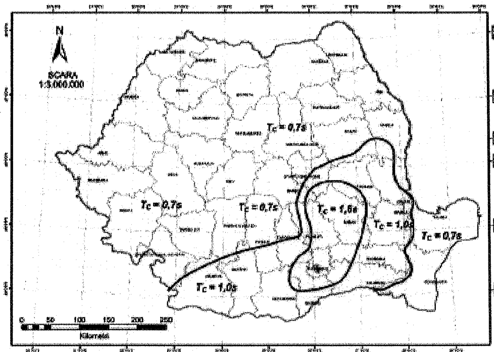
Figura 3: Zonarea teritoriului României în termeni de perioadă de control (colt), T_c a spectrului derăspuns, conform P100-1/2013 „Cod de proiectare seismică”
